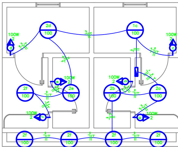
1 PLANTA BAIXA escala 1:50
