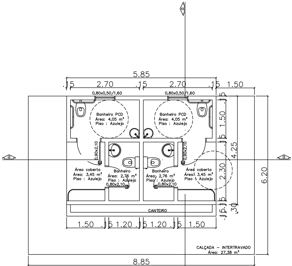
1 PLANTA BAIXA escala 1:50
