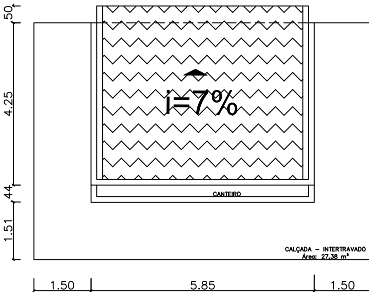
③ Planta de cobertura escala 1:75
